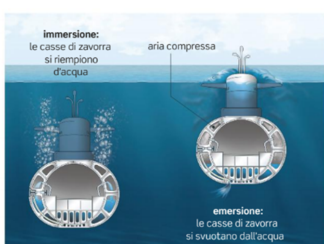
8 Funzionamento di un sommergibile.
